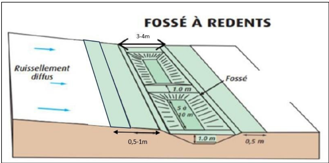
Dimensionnement d'un fossé à redents (source : Chambres d'Agriculture Seine-Maritime Eure / AREAS, modification Paysage 360)
