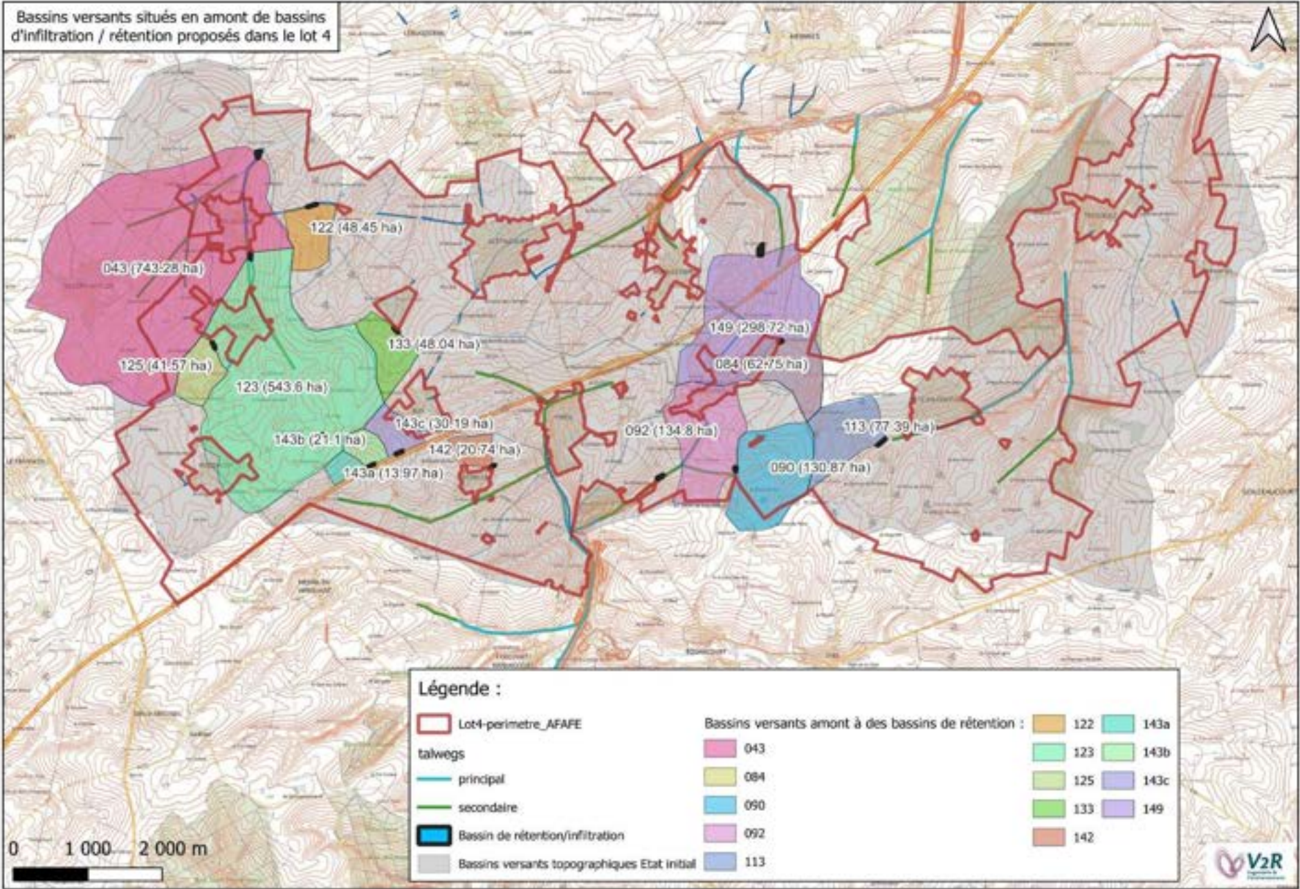
Carte de localisation des bassins-versants topographiques situés en amont de bassins d'infiltration/rétention proposés sur le secteur de l'AFAFE Lot 4 :
