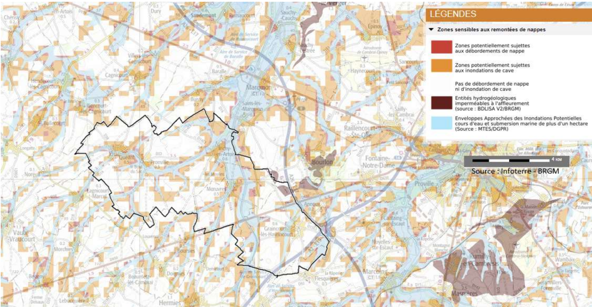
Risque remontée de la nappe phréatique
